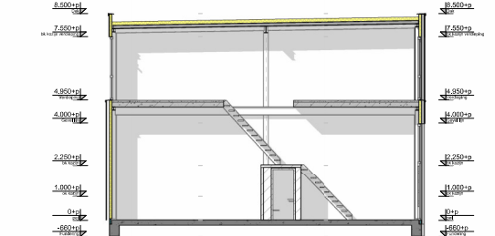
Doorsnede A
