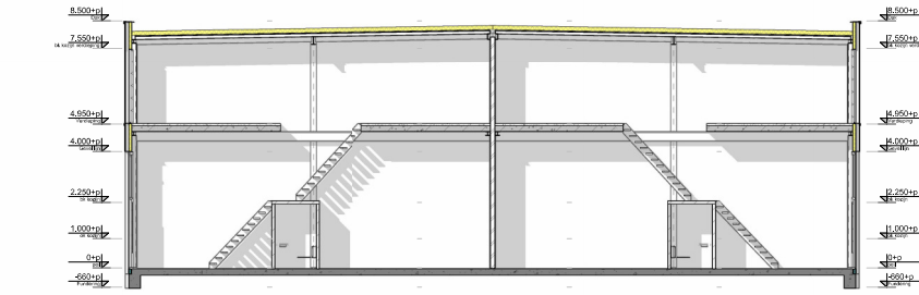
Doorsnede B
